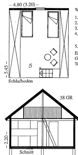
Schnitt
